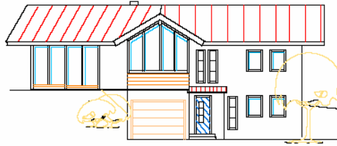
SÜDANSICHT
