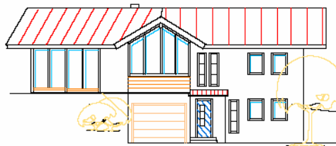
SÜDANSICHT
